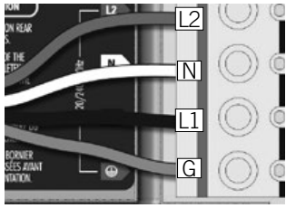
240 V (4 wires)
